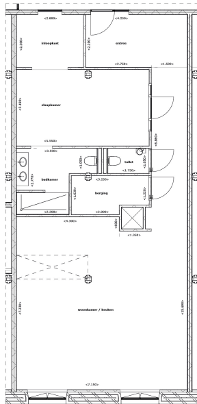
Plattegrond verdieping 02 1:50
