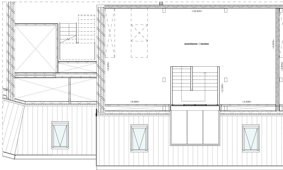
Plattegrond verdieping 04 1:50
