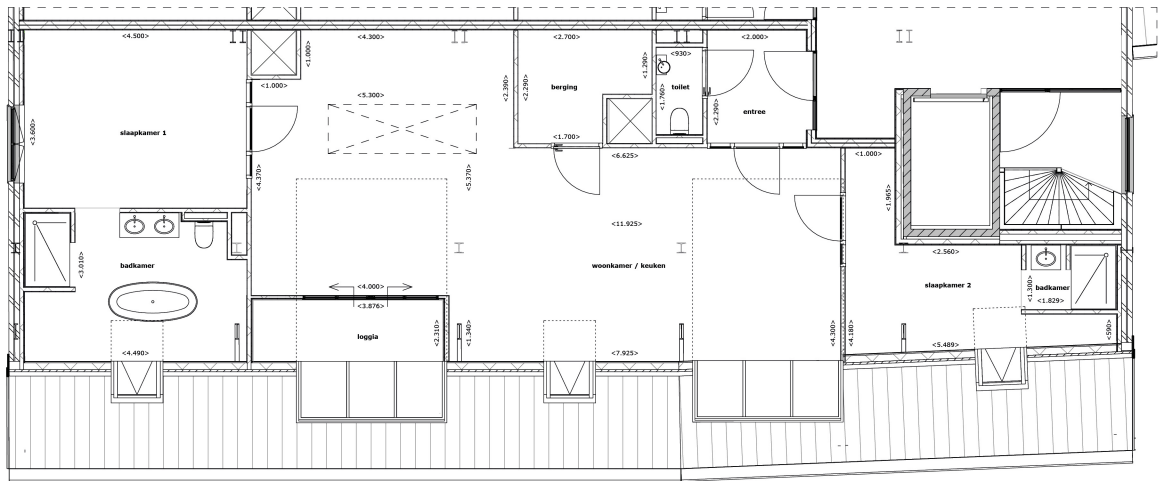
Plattegrond verdieping 04 1:50
